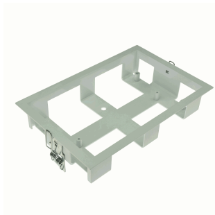
CADRE ENCASTREMENT PLAFOND / MURAL - DIM : 232X142X65mm - TOLEDO
