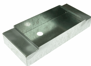
ACCESSOIRE ENCASTREMENT MURAL ( Plâtre , Ciment ) DIM : 336X145X61MM À associer avec un AMT0091
